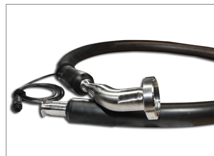
Et stort udvalg af Alfotech's fødevarer godkendte slanger kan monteres med el-tracing, samt med eller uden kontrol enhed. Slangerne overholder derfor gældende direktiver, som virksomhederne er pålagt. Eksempelvis produktioner af chokolade, fedt, honning etc.
